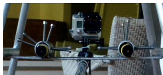
Figure 9: Photogrammetrie laser: une caméra entre deux lasers. Crédit photo: Nicolas Boudin.
