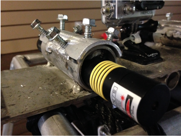
Figure 13: Tube en métal sur un BRUVS permettant le maintien et le calibrage d'un laser. Crédit photo: Nicolas Boudin.
